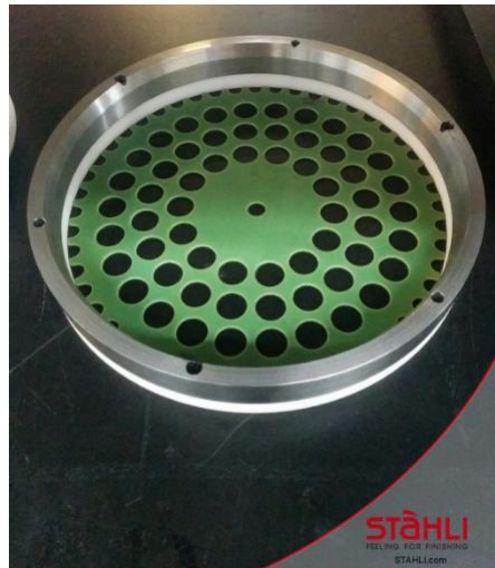
Image d'un satellite DLM 705 dans un anneau de dressage FH 702-H
